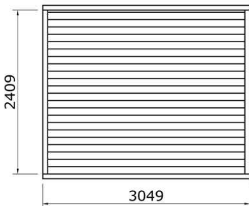
Bovenaanzicht
