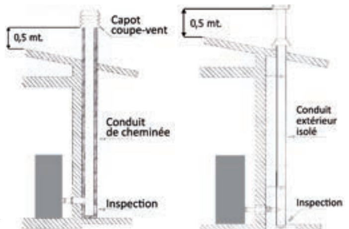
Fig. 2: raccord au conduit de cheminée
