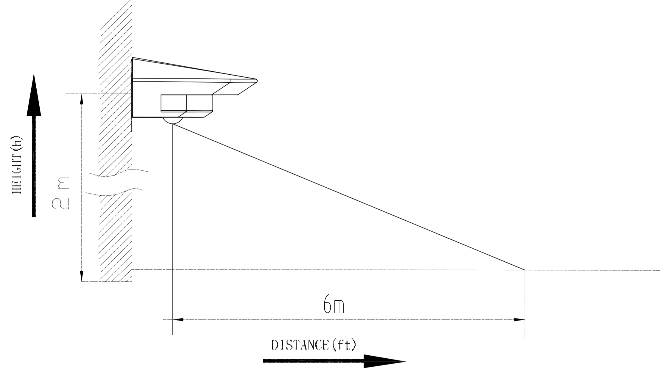
当灯的高度装在离地2.m高时，感应距离达到最远6m
