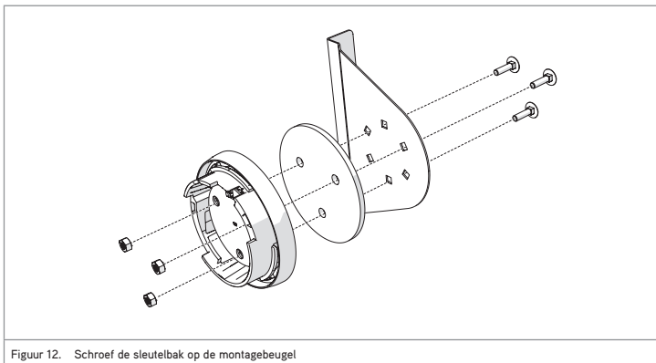
Figuur 12. Schroef de sleutelbak op de montagebeugel
