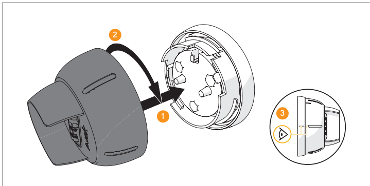
Figuur 11. Plaats de deksel
