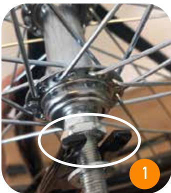
Voorvork
