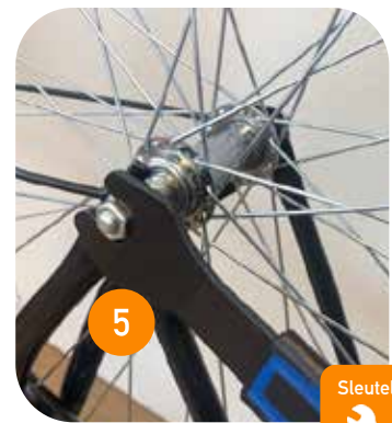
Vastdraaien
