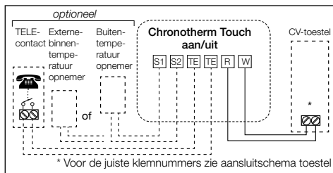
Figuur 6: Aansluitschema
